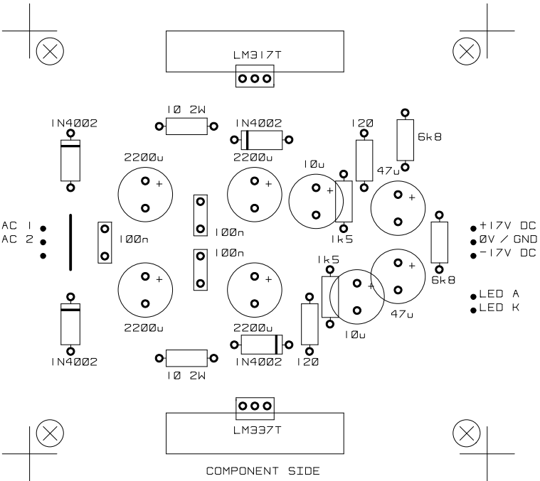
VI.1 AC PLUGPACK VERSION
